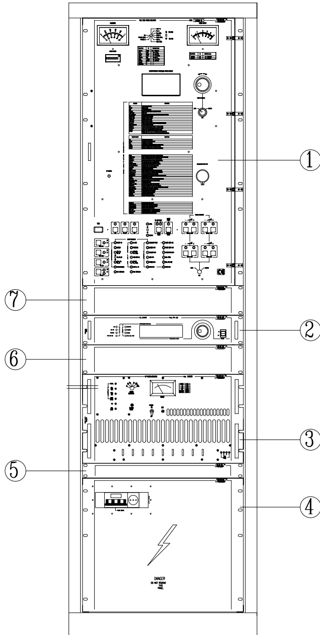
FIGURA 1 VISTA FRONTALE
